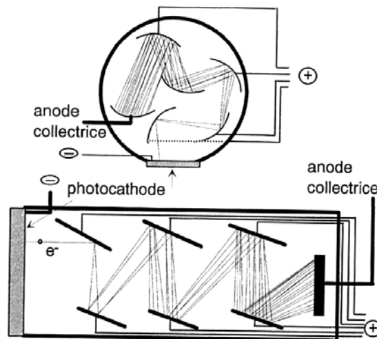
Figure III-6. Les photomultiplicateurs.
