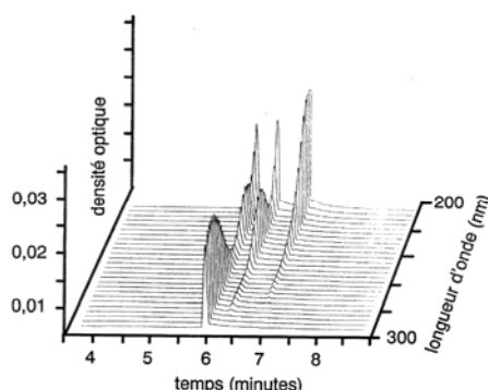
Figure VI-24 : Profil d'élution tridimensionnel en HPLC, obtenu grâce à un détecteur photométrique à barrette de diodes.
