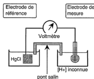
Figure IV-3 : Principe de la mesure du pH à l'aide d'électrodes n'utilisant pas l'hydrogène.
