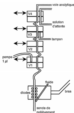
Figure V-14 : Les électrovannes à segmentation du Chem 1.
