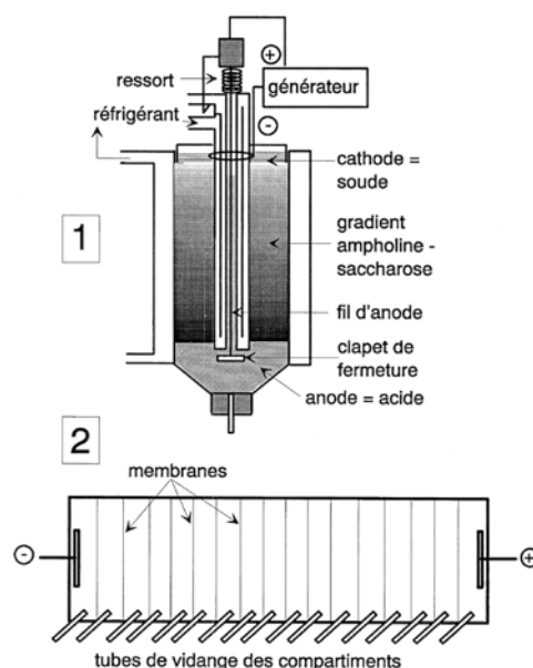
Figure VI-32 : Systèmes d'électrofocalisation en veine liquide.
