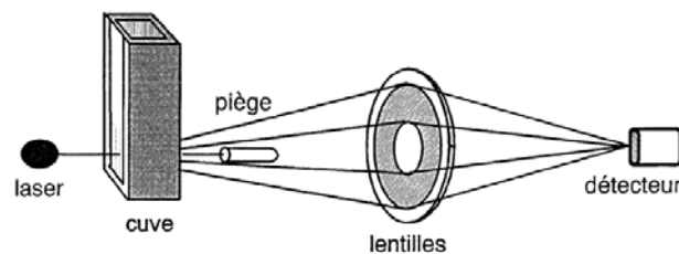
Figure III-24. Néphélométrie laser avec mesure selon un angle solide.
