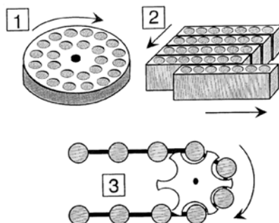
Figure V-7 : Les systèmes de positionnement des échantillons.
