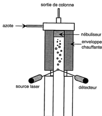
Figure VI-25 : Détecteur HPLC à diffusion de lumière après évaporation (ELSD).
