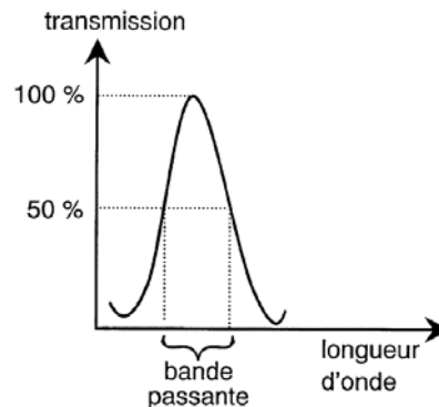
Figure III-4. Définition de la largeur de la bande passante d'un filtre.
