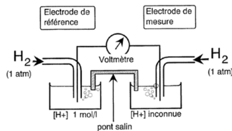
Figure IV-2 : Mesure du pH à l'aide d'électrodes à hydrogène.
