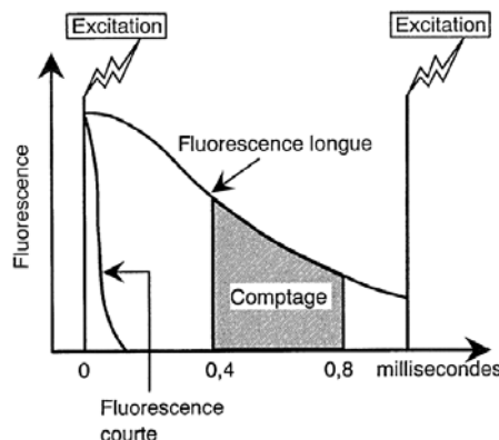
Figure III-23. Principe de la mesure de fluorescence en temps résolu.
