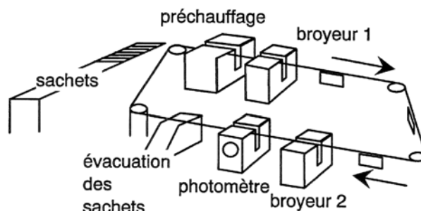
Figure V-25 : Principe d'organisation de l'automate ACA.
